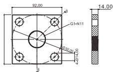
Flange
